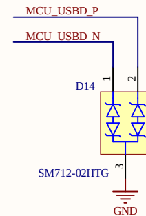
TVS USB DATA
